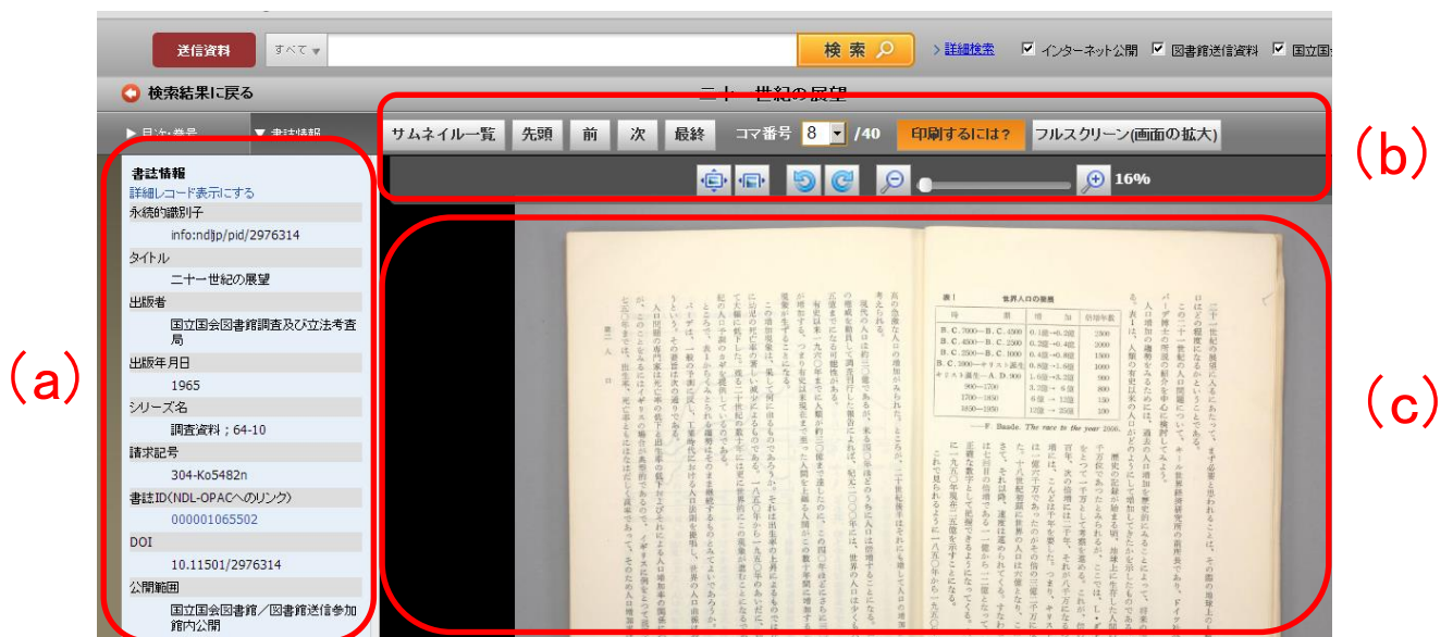
図 3-1 閲覧画面
